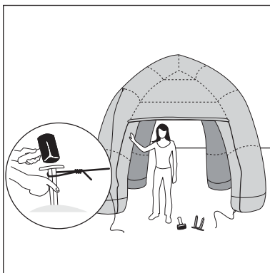
SICHERN DES ZELTES
